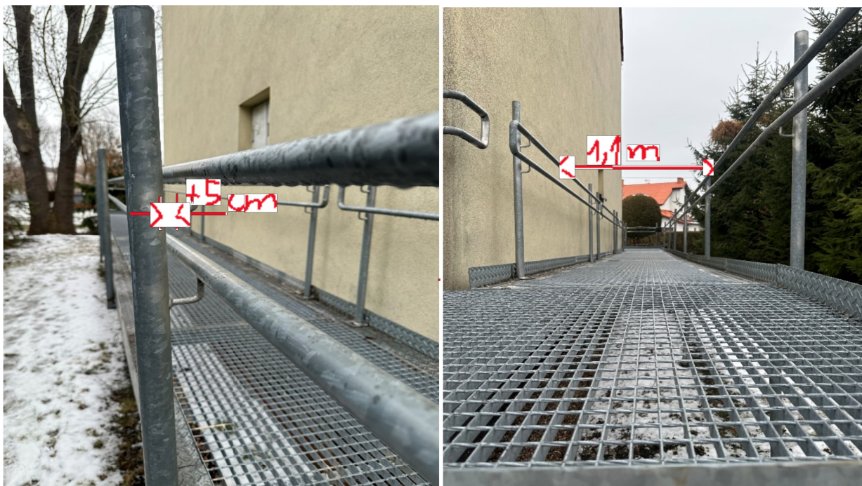
Zdjęcie nr 5 i 6. Korekcja odległości pomiędzy dwupoziomowymi pochwytyami na całym odcinku pochylni.
